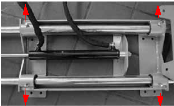
Fig. 11 Onderkant met juist uitgelijnde smeernippels
