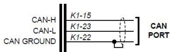
Cableado de la red de la CAN
